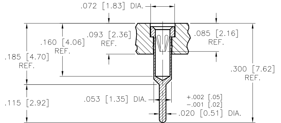
SECTION A-A -01S
